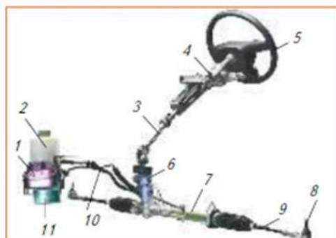
Рис. 4.3. Подсистема рулевого управления: 1 — электронный блок управления; 2 — бачок с жидкостью; 3 — карданный вал; 4 — рулевая колонка; 5 — рулевое колесо; 6 — распределитель жидкости; 7 — блок цилиндров; 8 — наконечник рулевой тяги с шаровым шарниром для поворота колеса; 9 — рулевая тяга; 10 — шланги; 11 — насос с электродвигателем
