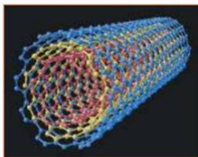
Рис. 14.5. Нанообъекты
